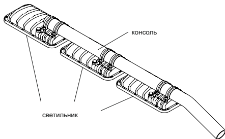
Рисунок 2 – Установка нескольких светильников на одну консоль
