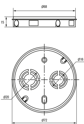
Коробка установочная KMT-194
