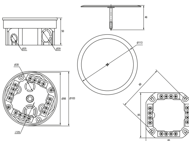
Коробка установочная KMT-010-021
