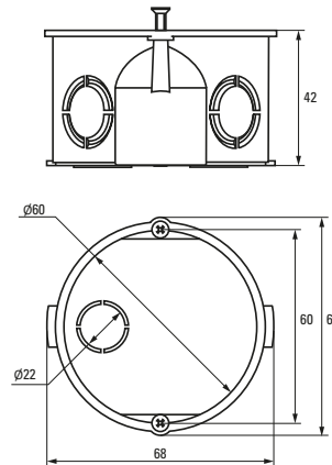
Коробка установочная KMT-010-003
