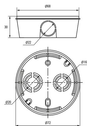
Коробка установочная KMT-195
