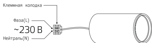
Рис. 1. Схема подключения к электросети 230 В
