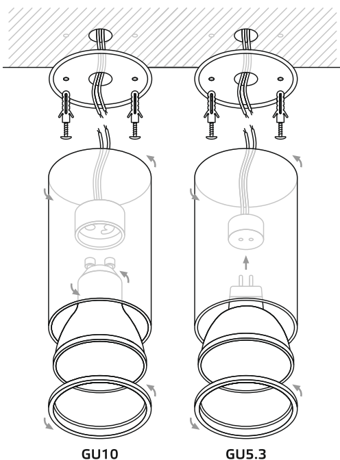
Рис. 2. Порядок монтажа
